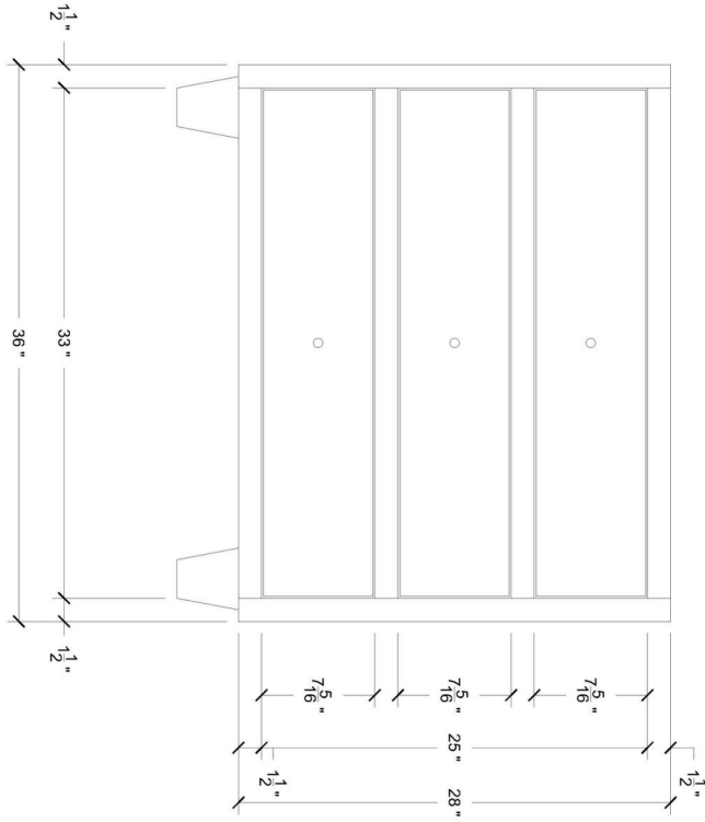
1 FRONT ELEVATION 01 Scale: 1" = 10"
